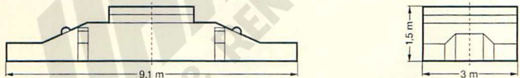
Raupennittelteil / Crawler center frame / Partie centrale
